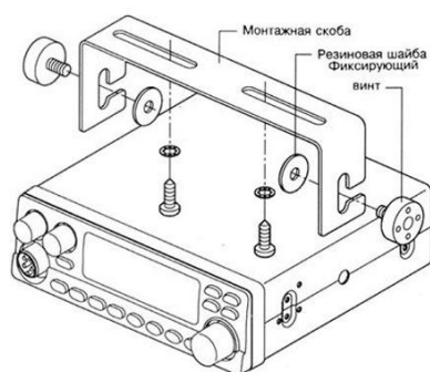
Рис.1. Крепление радиостанции при помощи монтажной скобы.
